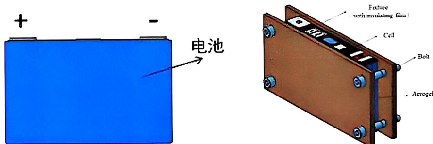
图2 夹具安装示意图 Fixture tools assembly diagram
