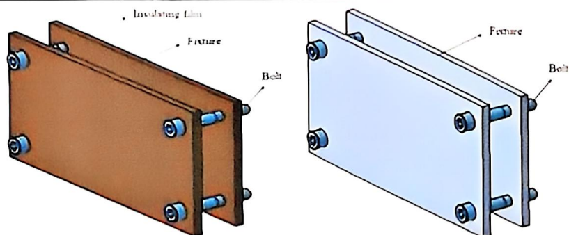
图1 电池测试夹具示意图 Cell testing fixture diagram
