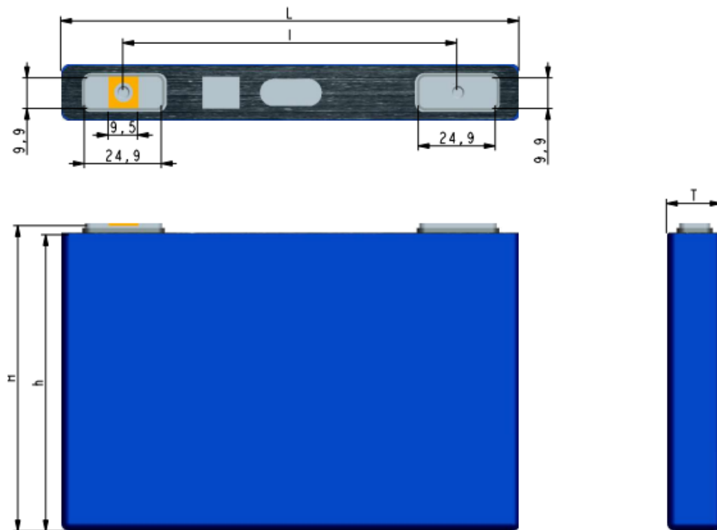
图 1 INP20P 外形尺寸图
