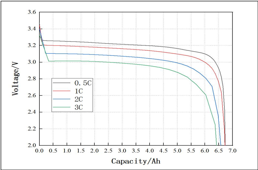
6.7Ah 磷酸铁锂系电池不同倍率放电曲线 Different rate discharge curve of 6.7Ah LiFePO 4 cell
