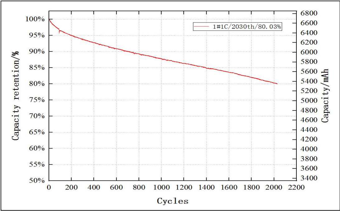
6.7 Ah 磷酸铁锂电池 30±2℃ 1C 循环曲线图 30±2℃ 1C cycle curve of 6.7Ah LiFePO 4 cell
